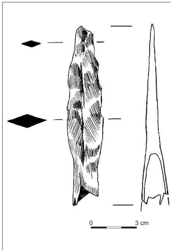
Ryc. 2. Żelazny grot oszczepu z Bojszowa. Rys. R. Polackiewicz.
