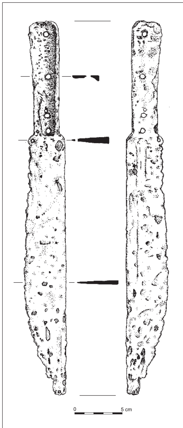
Ryc. 1. Burdze, pow. stalowowolski. Późnośredniowieczny puginał nożowy. Rys. P. N. Kotowicz, przerys A. Sabat.
